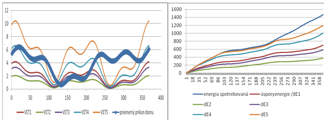
Obrázok 7 Porovnanie príkonu a spotreby budovy a využiteľný výkon a ušetrená energia
